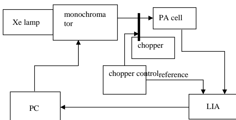
Figure 1 PAS system
