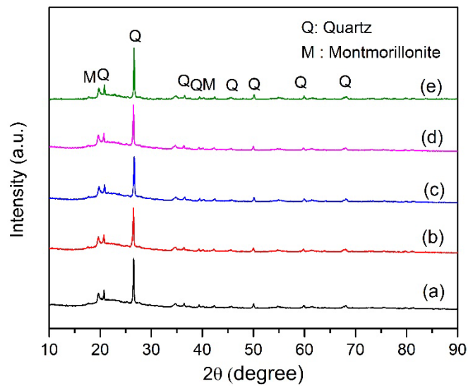
Figure 4. XRD patterns of DE with gamma radiation dose levels: (a) DE, (b) DE 5 kGy, (c) DE 10 kGy, (d) DE 20 kGy and (e) DE 30 kGy
