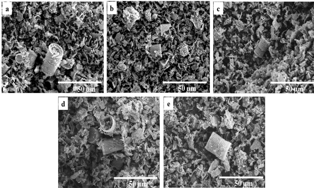
Figure 3. FE-SEM of DE with gamma radiation dose levels (a) DE, (b) DE 5 kGy, (c) DE 10 kGy, (d) DE 20 kGy and (e) DE 30 kGy
