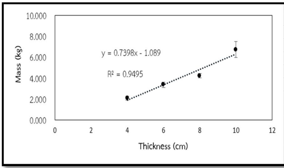
ภาพที่ 5 กราฟความสัมพันธ์ระหว่างความหนาและมวลที่ทำให้แพจมพอดี จากการคำนวณ
