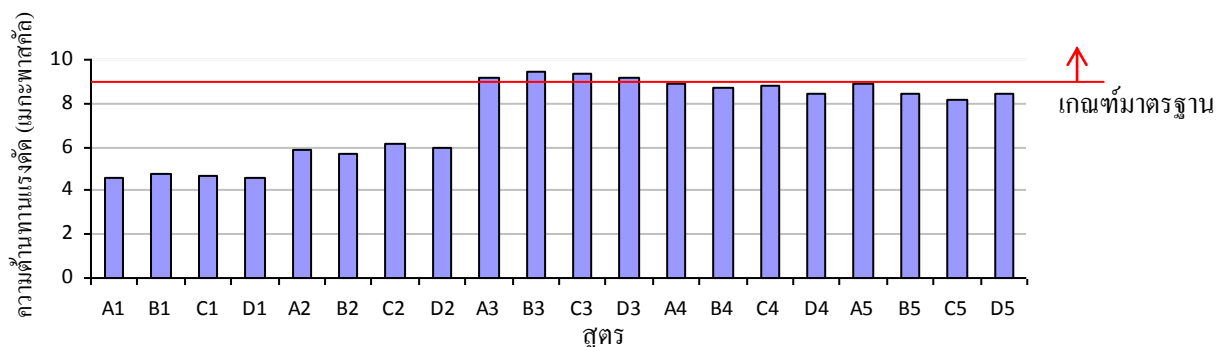
ภาพที่ 9 ผลการทดสอบความต้านทานแรงอัดของแผ่นใยอัดซีเมนต์ผสมเส้นใยผักตบชวา
