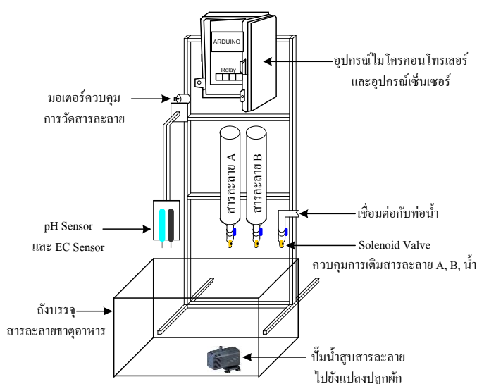
ภาพที่ 5 ชุดอุปกรณ์วัดค่าสารละลายธาตุอาหารสำหรับปลูกผักไฮโดรโปนิกส์
