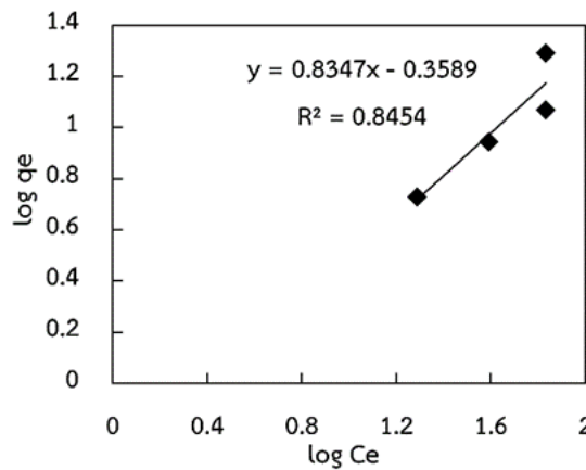
ภาพที่ 9 ไอโซเทอร์มการดูดซับ COD ด้วยถ่านลอยจากโรงงานสกัดน้ำมันปาล์มโดยใช้สมการการดูดซับของฟรุนดิช
