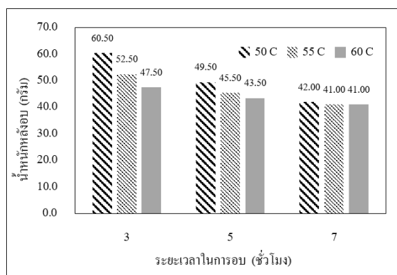
ภาพที่ 5 กราฟแสดงอัตราส่วนการอบแห้งของสมุนไพรใบพลู
