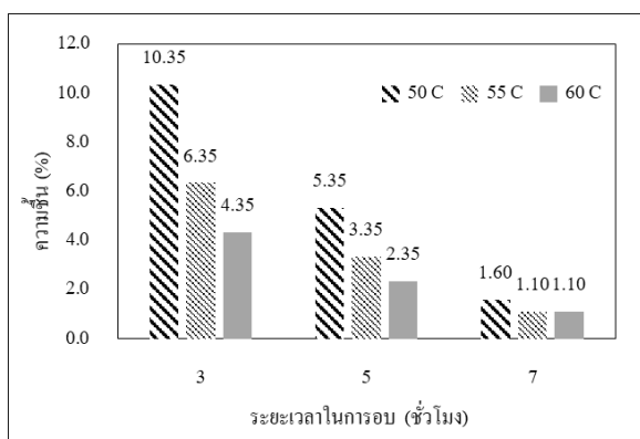
ภาพที่ 3 กราฟแสดงผลความชื้นหลังการอบสมุนไพรใบพลู
