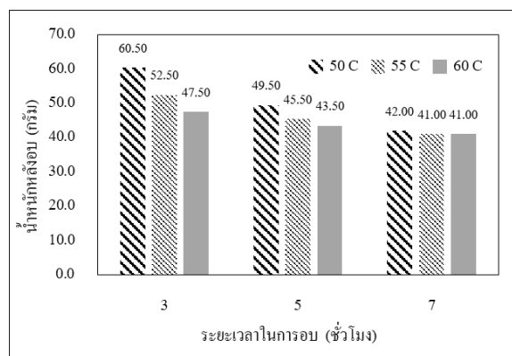
ภาพที่ 4 กราฟแสดงผลน้ำหนักหลังการอบสมุนไพรใบพลู
