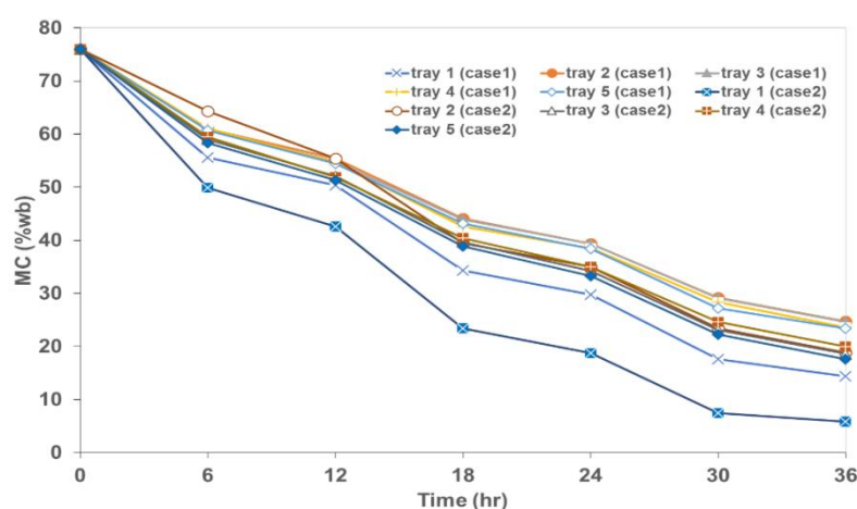
ภาพที่ 8 ความชื้นของผลิตภัณฑ์แต่ละถาดกับเวลา ระบบบอบแห้งด้วยปั๊มความร้อนร่วมรังสีอาทิตย์แบบเรือนกระจก กรณีไม่มีเรือนกระจก (case 1) กับติดตั้งเรือนกระจก (case 2)
