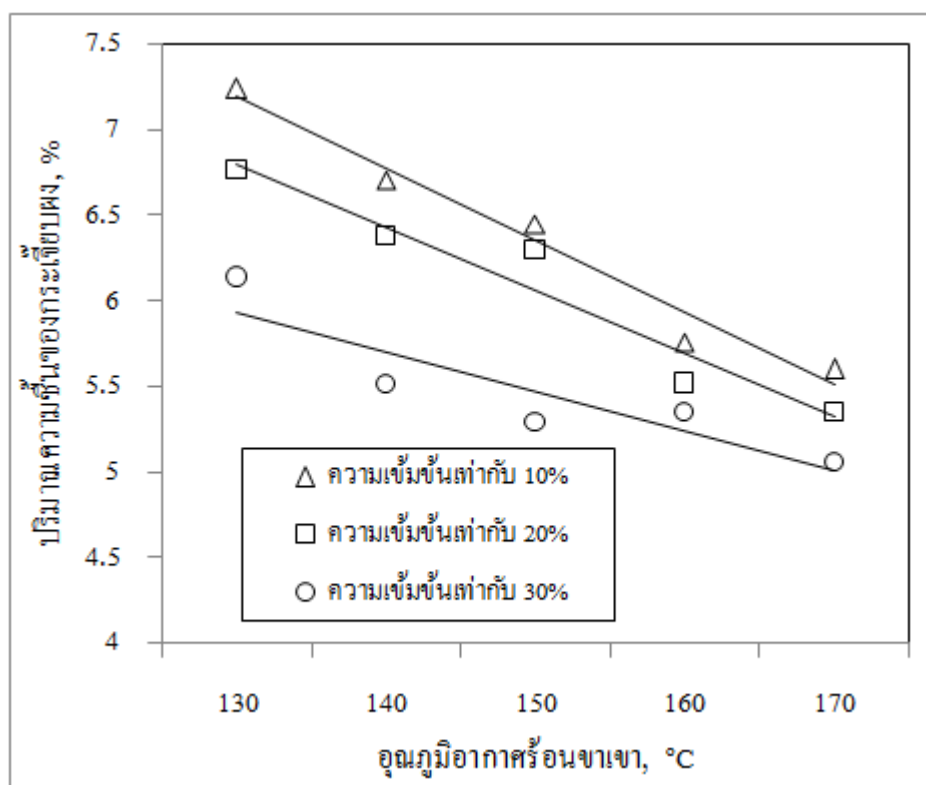
ภาพที่ 3 ความสัมพันธ์ระหว่างอุณหภูมิอากาศร้อนขาเข้ากับความชื้นของสารละลายต่างๆ ที่อัตราการไหลของอากาศ 0.0410 \text{ m}^3/\text{s} (วสันต์, 2546)
