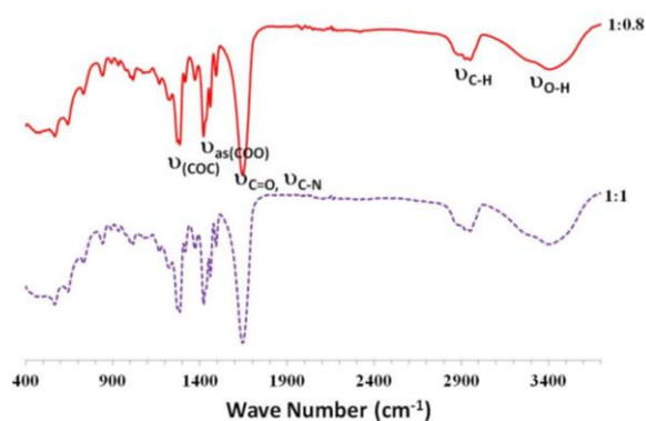
ภาพที่ 3 FT-IR spectrum สำหรับไฮโดรเจลที่สังเคราะห์ได้จากเพคตินของผลชาว์บันพระฤๅษีและ PVP
