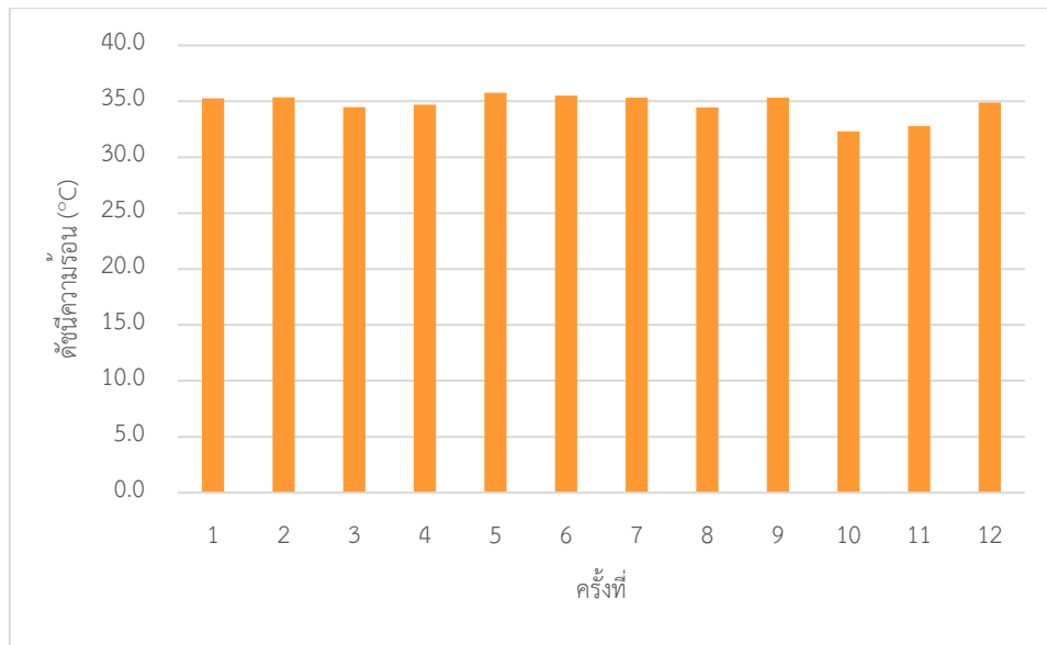
ภาพที่ 7 กราฟแสดงดัชนีความร้อนของการทำงานในตู้แช่สมรรถยนต์ขนาดใหญ่
