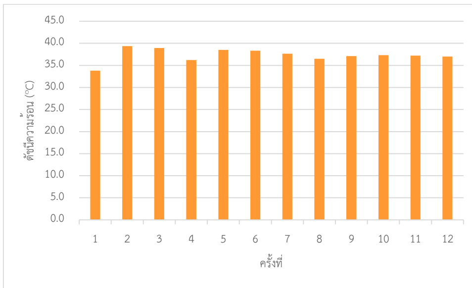
ภาพที่ 8 กราฟแสดงดัชนีความร้อนของการทำงานในตู้แช่สมรรถยนต์ขนาดเล็ก
