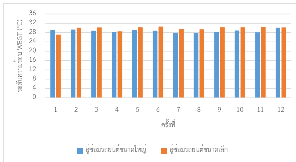
ภาพที่ 11 กราฟแสดงระดับความร้อนของการทำงานของอุณหภูมิห้องขนาดใหญ่และขนาดเล็ก
