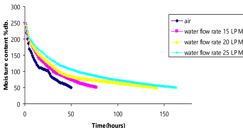
ภาพที่ 5 แสดงการเปลี่ยนแปลงความชื้นมาตรฐานแห้งในไม้ในการผลิตเครื่องดนตรีอีสาน (ไม้ต้นรักใหญ่) เทียบกับเวลา
