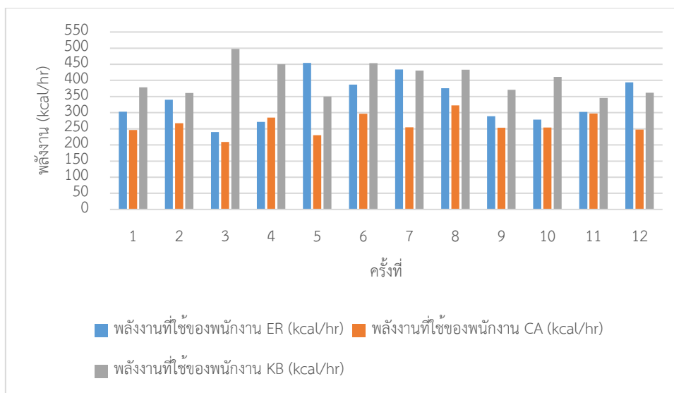
ภาพที่ 9 กราฟแสดงพลังงานที่ใช้ของผู้ปฏิบัติงานในอุโมงค์มรณต์ขนาดใหญ่
