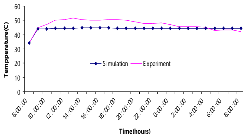
ภาพที่ 23 แสดงเปรียบเทียบอุณหภูมิอากาศที่ทางออกตู้อบแห้งอัตราการไหลของอากาศ 2.13 กิโลกรัมต่อวินาที
