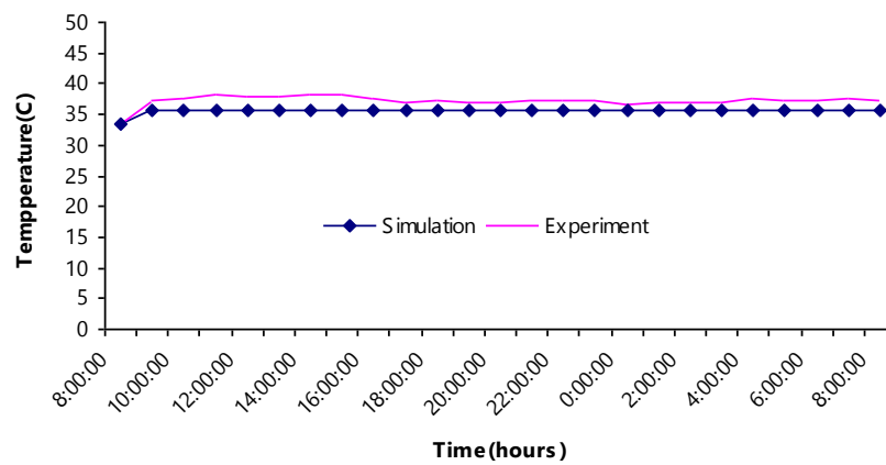
ภาพที่ 15 แสดงการเปรียบเทียบอุณหภูมิน้ำที่ทางออกของอุปกรณ์แลกเปลี่ยนความร้อนภายในตู้อบแห้ง อัตราการไหลของน้ำ 20 ลิตรต่อนาที
