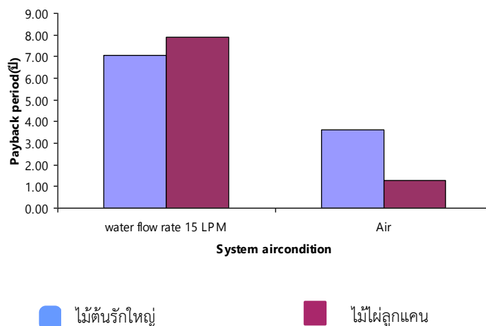
ภาพที่ 25 เปรียบเทียบระยะเวลาในการคืนทุนของการอบแห้งในระบบปรับอากาศแบบระบายความร้อนด้วยน้ำ และระบายความร้อนด้วยอากาศ
