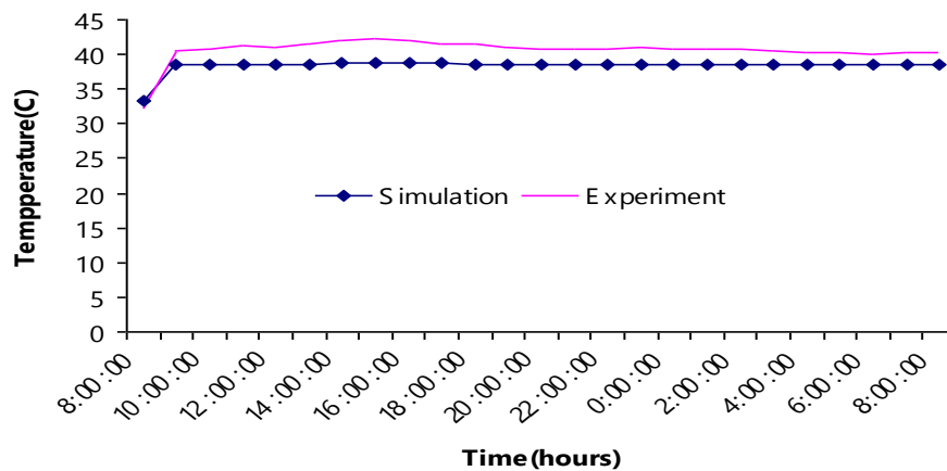
ภาพที่ 11 แสดงการเปรียบเทียบอุณหภูมิที่ทางออกของอุปกรณ์แลกเปลี่ยนความร้อนภายในตู้อบแห้ง อัตราการไหลของน้ำ 15 ลิตรต่อนาที
