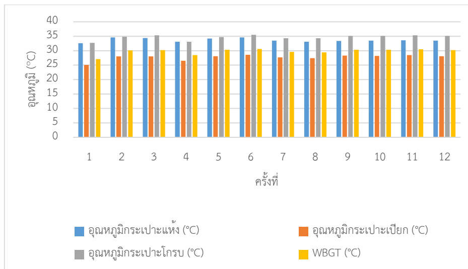
ภาพที่ 2 กราฟแสดงระดับความร้อนของการทำงานในอุโมงค์รถยนต์ขนาดเล็ก
