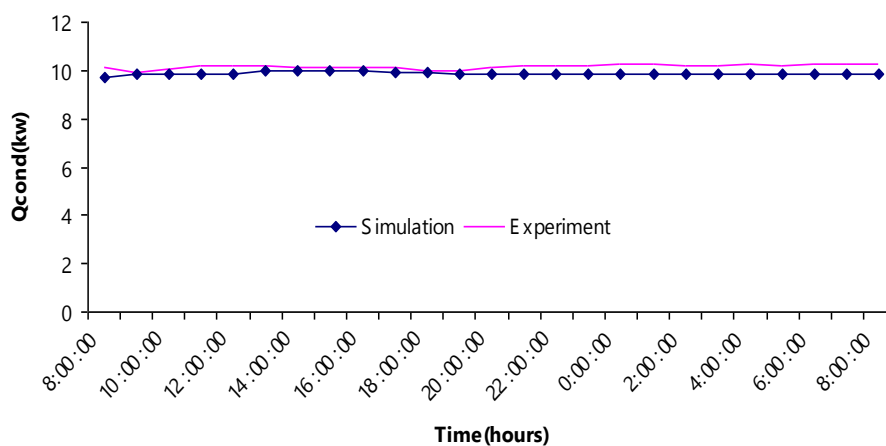
ภาพที่ 9 แสดงการเปรียบเทียบอัตราการถ่ายเทความร้อนของคอนเดนเซอร์ที่ระบายความร้อนด้วยน้ำ อัตราการไหลของน้ำ 15 ลิตรต่อนาที
