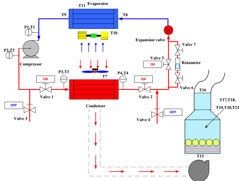
ภาพที่ 1 แสดงแผนผังแสดงการทำงานของระบบปั๊มความร้อน (Heat Pump System) ที่นำความร้อนทิ้งจากส่วนคอยล์ร้อน (Condenser) มาใช้ประโยชน์ในการอบแห้งหรือทำความร้อน
