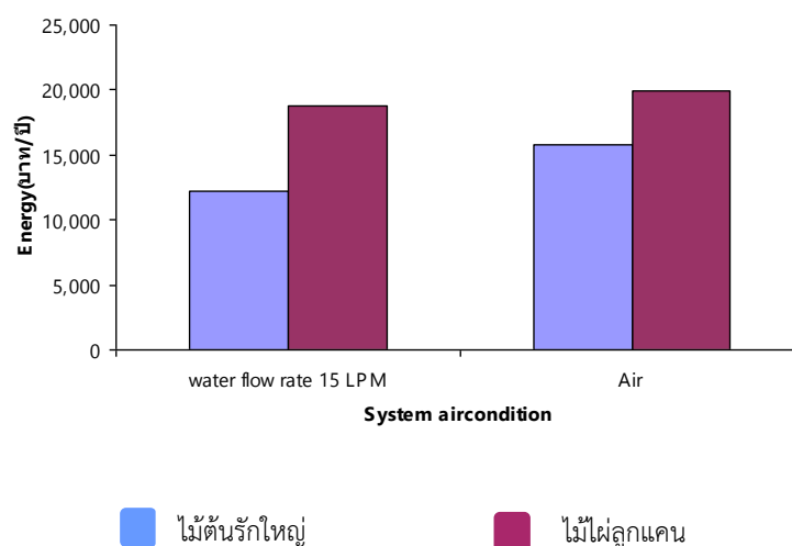
ภาพที่ 24 เปรียบเทียบพลังงานที่ใช้ในการอบแห้งในระบบปรับอากาศแบบระบายความร้อนด้วยน้ำ และระบายความร้อนด้วยอากาศ
