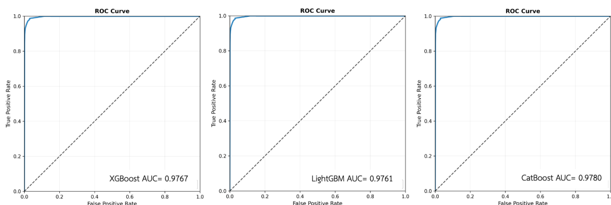
ภาพที่ 5 แสดงการเปรียบเทียบประสิทธิภาพแบบจำลองด้วยการวิเคราะห์กราฟพื้นที่ใต้เส้นโค้งอาร์โอซี
