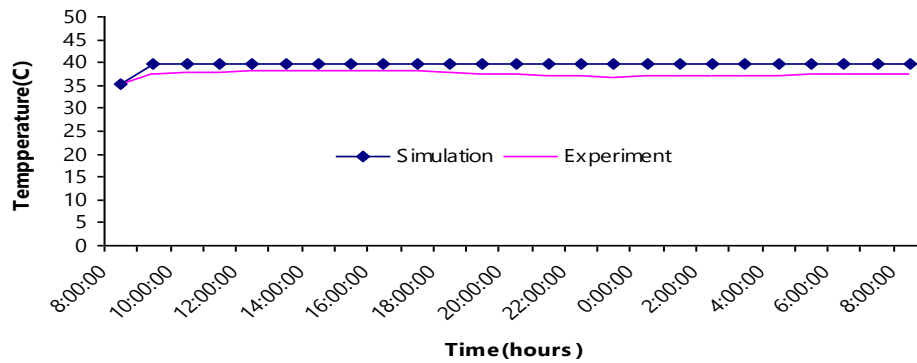
ภาพที่ 20 แสดงการเปรียบเทียบอุณหภูมิอากาศที่ทางออกของอุปกรณ์แลกเปลี่ยนความร้อนภายในตู้อบแห้งอัตราการไหลของน้ำ 25 ลิตรต่อวินาที อัตราการไหลของอากาศ 2.13 กิโลกรัมต่อวินาที
