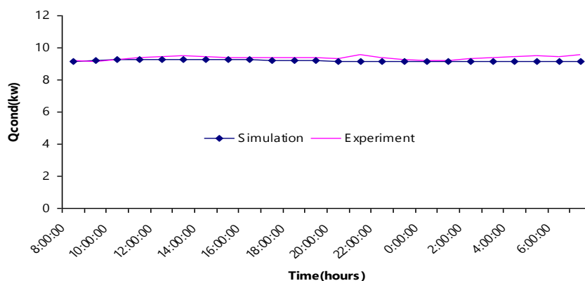
ภาพที่ 13 แสดงการเปรียบเทียบอัตราการถ่ายเทความร้อนของคอนเดนเซอร์ที่ระบายความร้อนด้วยน้ำ อัตราการไหลของน้ำ 20 ลิตรต่อนาที
