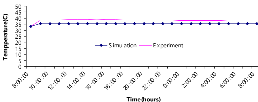
ภาพที่ 19 แสดงการเปรียบเทียบอุณหภูมิน้ำที่ทางออกของอุปกรณ์แลกเปลี่ยนความร้อนภายในตู้อบแห้งอัตราการไหลของน้ำ 25 ลิตรต่อนาที
