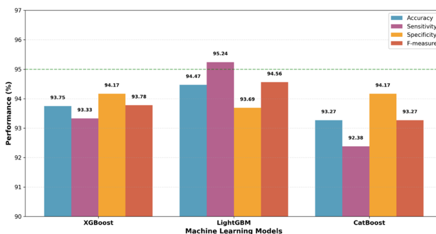
ภาพที่ 4 แสดงการเปรียบเทียบประสิทธิภาพแบบจำลองการเรียนรู้ของเครื่องแบบบูสต์
