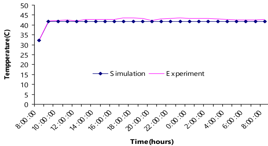
ภาพที่ 10 แสดงการเปรียบเทียบอุณหภูมิที่ทางออกของคอนเดนเซอร์ที่ระบายความร้อนด้วยน้ำ อัตราการไหลของน้ำ 15 ลิตรต่อนาที
