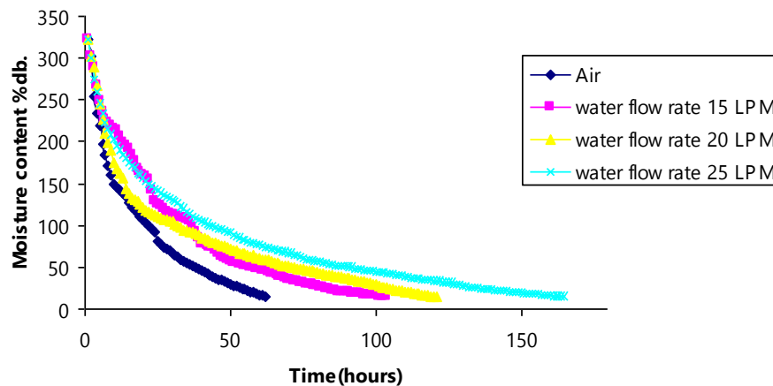
ภาพที่ 7 แสดงการเปลี่ยนแปลงความชื้นมาตรฐานแห้งในไม้ในการผลิตเครื่องดนตรีอีสาน (ไผ่ลูกแคน) เทียบกับเวลา
