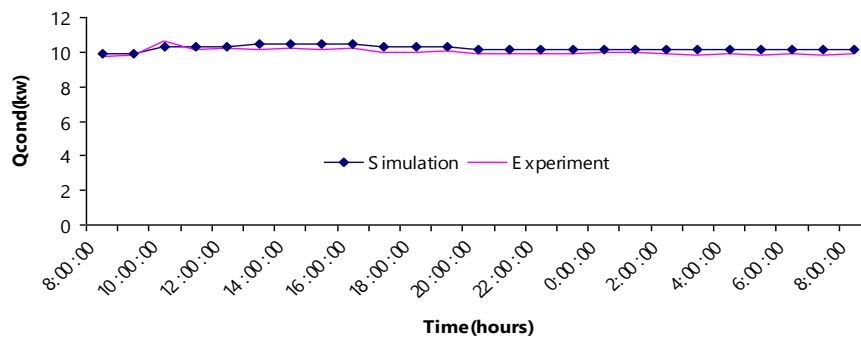
ภาพที่ 21 แสดงการเปรียบเทียบอัตราการถ่ายเทความร้อนของคอนเดนเซอร์ที่ระบายความร้อนด้วยอากาศอัตราการไหลของอากาศ 0.90 กิโลกรัมต่อวินาที
