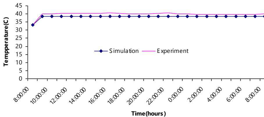
ภาพที่ 18 แสดงการเปรียบเทียบอุณหภูมิน้ำที่ทางออกของคอนเดนเซอร์ที่ระบายความร้อนด้วยน้ำอัตราการไหลของน้ำ 25 ลิตรต่อนาที
