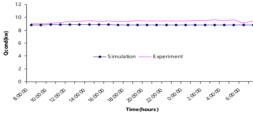
ภาพที่ 17 แสดงการเปรียบเทียบอัตราการถ่ายเทความร้อนของคอนเดนเซอร์ที่ระบายความร้อนด้วยน้ำอัตราการไหลของน้ำ 25 ลิตรต่อนาที
