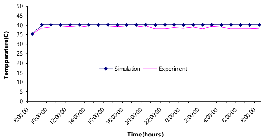
ภาพที่ 16 แสดงการเปรียบเทียบอุณหภูมิอากาศที่ทางออกของอุปกรณ์แลกเปลี่ยนความร้อนภายในตู้อบแห้ง อัตราการไหลของน้ำ 20 ลิตรต่อนาที อัตราการไหลของอากาศ 2.13 กิโลกรัมต่อวินาที
