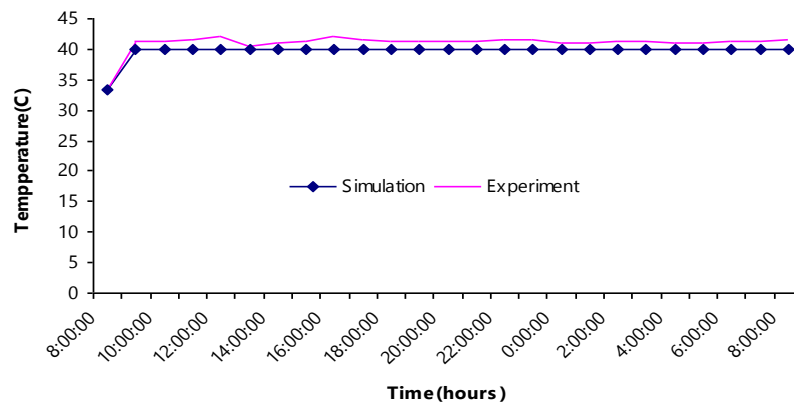
ภาพที่ 14 แสดงการเปรียบเทียบอุณหภูมิน้ำที่ทางออกของคอนเดนเซอร์ที่ระบายความร้อนด้วยน้ำ อัตราการไหลของน้ำ 20 ลิตรต่อนาที
