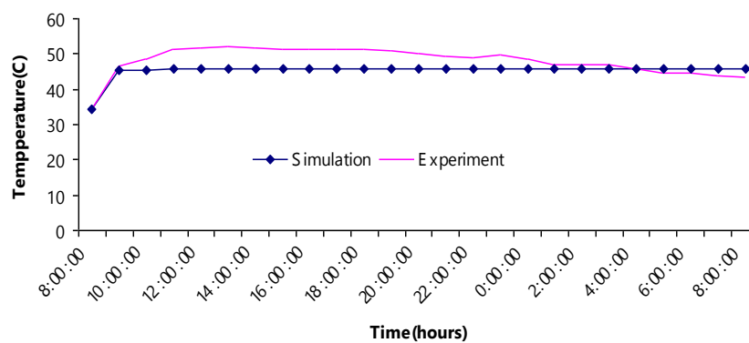
ภาพที่ 22 แสดงการเปรียบเทียบอุณหภูมิอากาศที่ทางออกของคอนเดนเซอร์อัตราการไหลของอากาศ 0.90 กิโลกรัมต่อวินาที
