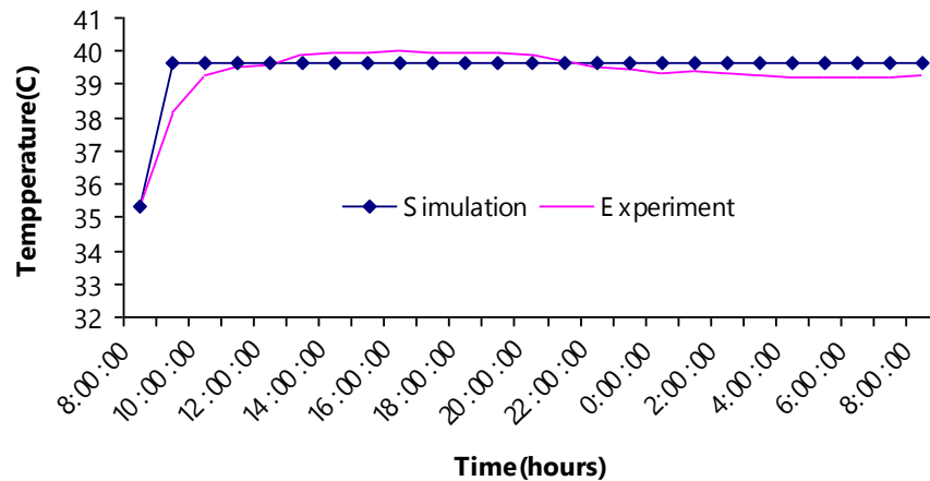
ภาพที่ 12 เปรียบเทียบอุณหภูมิอากาศที่ทางออกของอุปกรณ์แลกเปลี่ยนความร้อนภายในตู้อบแห้งอัตราการไหลของน้ำ 15 ลิตรต่อนาที อัตราการไหลของอากาศ 2.13 กิโลกรัมต่อวินาที
