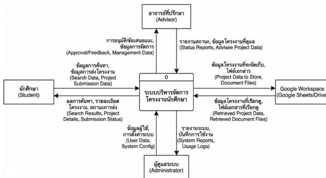
ภาพที่ 2 แผนภาพบริบท (Context Diagram) ของระบบ
