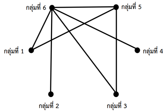
ภาพที่ 12 กราฟปัญหาการจัดตารางประชุม
