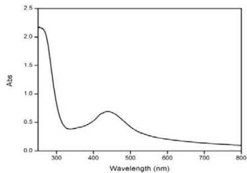
รูปที่ 5 สเปกตรัมการดูดกลืนแสงของแผ่นฟิล์มโพลิเมอร์ไอโบลิตไวแสงซิลิกอนไดออกไซด์และไทเทเนียมไดออกไซด์
