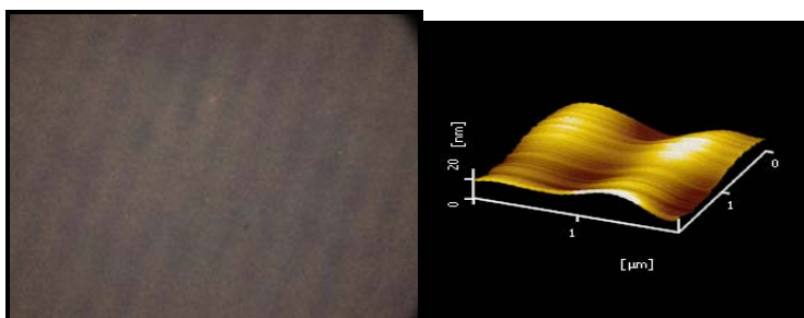
รูปที่ 7 ลวดลายของเกรตติงเลี้ยวเบน (ก) กล้องจุลทรรศน์แบบแสง (ข) กล้องจุลทรรศน์แรงอะตอม
