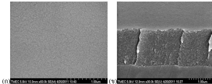
รูปที่ 4 ลักษณะของแผ่นฟิล์มไฮบริดไวแสงซิลิกอนไดออกไซด์และไทเทเนียมไดออกไซด์ (ก) พื้นผิว (ข) ภาพตัดขวาง
