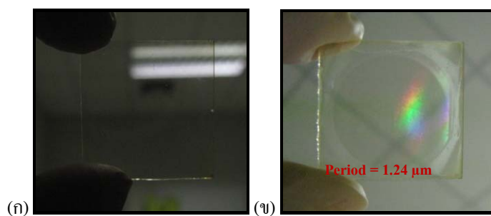
รูปที่ 6 ฟิล์มโพลิเมอร์ไอโบลิตไวแสง (ก) ก่อนและ (ข) หลังผ่านการฉายด้วยแสงเลเซอร์โดยผ่านกระบวนการล้างด้วยเอทานอล
