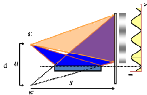
รูปที่ 2 ระบบการแทรกสอดของแสงเลเซอร์โดยใช้กระจกของลอยด์
