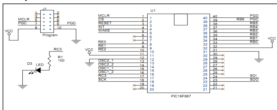
รูปที่ 7 วงจรควบคุมการทำงาน
