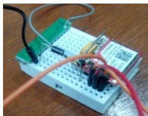
รูปที่ 4. การประกอบ SIM800L เข้ากับ Breadboard
