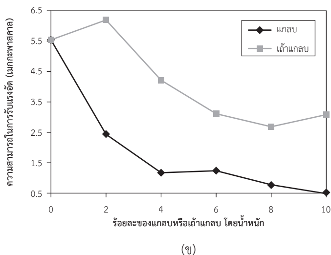
ภาพที่ 2 กราฟความสัมพันธ์ระหว่างส่วนผสมกับ (ก) ความหนาแน่นของอิฐมอดู (ข) ความสามารถในการรับแรงอัด
