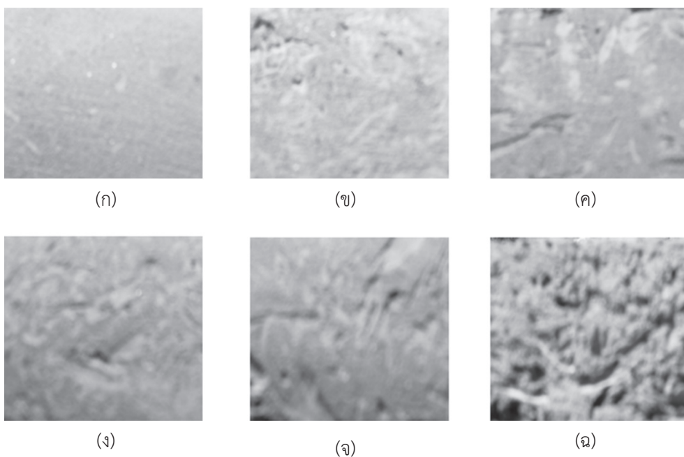
ภาพที่ 4 ภาพถ่ายภาคตัดขวางของอิฐมอญที่ส่วนผสมของดินต่อแกลบที่ปริมาณร้อยละ (ก) 0, (ข) 2, (ค) 4, (ง) 6 (จ) 8, (ฉ) 10 โดยน้ำหนัก
