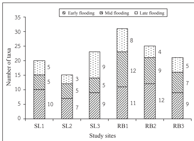
ภาพที่ 2 จำนวนวงศ์ของแมลงน้ำในนาข้าวทั้ง 6 แปลงในช่วง 1 ฤดูกาลทำนา
