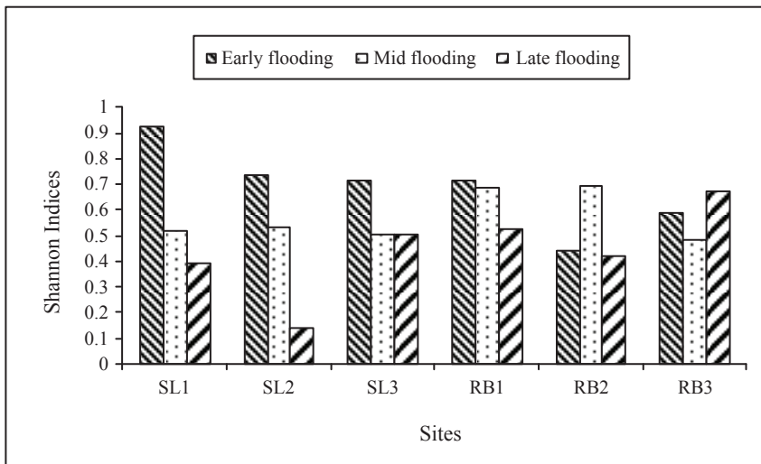
ภาพที่ 4 ดัชนีความหลากหลายของแมลงน้ำในนาข้าวแต่ละแปลงในช่วง 1 ฤดูกาลทำนา
