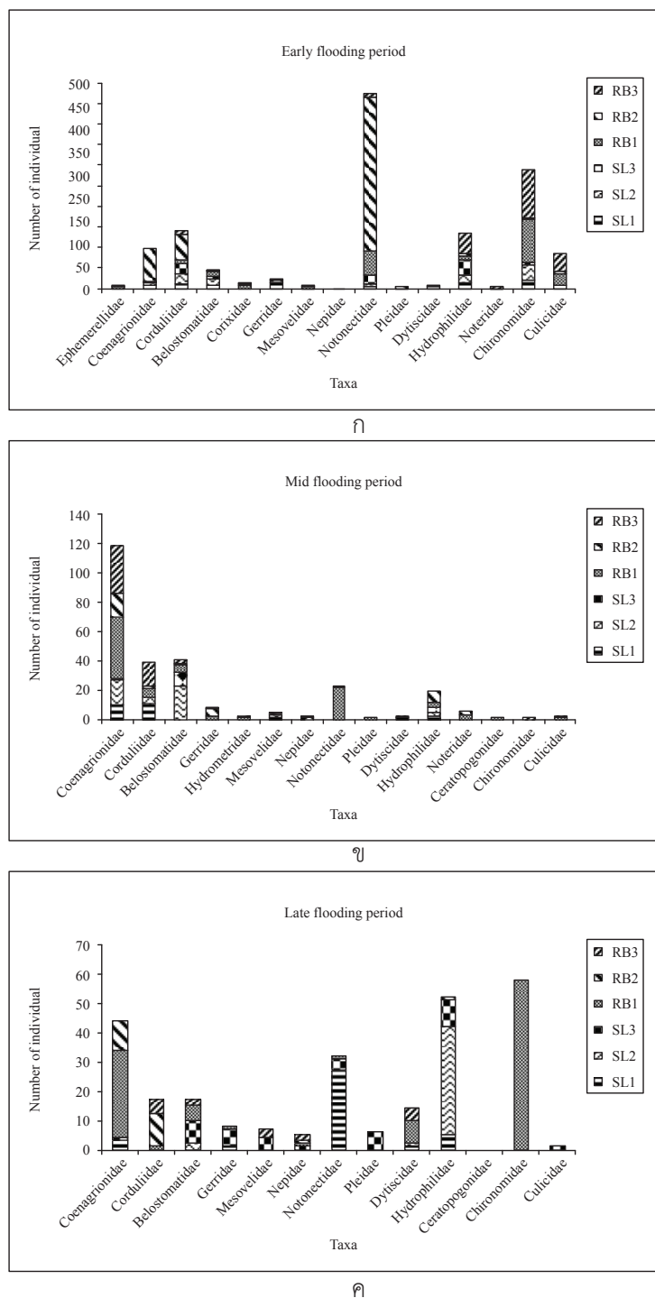
ภาพที่ 3 จำนวนตัวทั้งหมดของแมลงน้ำในแต่ละวงศ์ที่พบในนาข้าว ก) ช่วงแรกของการทำนา ข) ช่วงกลางของการทำนา ค) ช่วงท้ายของการทำนา
