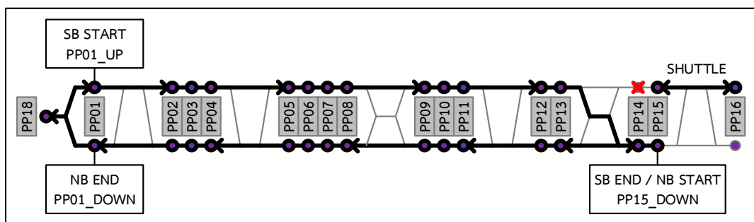
รูปที่ 2 รูปแบบการเดินทางไฟฟ้าสภาวะไม่ปกติในสถานการณ์ที่ 3
