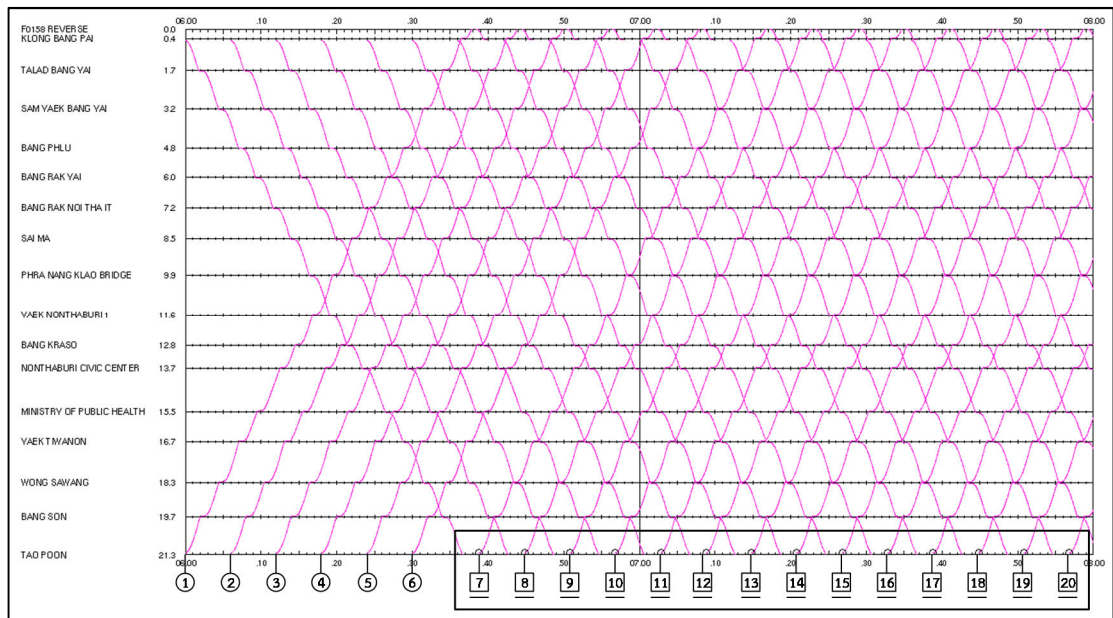
รูปที่ 4 ผังการเดินทางแสดงความล่าช้าในการออกรถจากสถานีเตาปูนกรณีปล่อยรถพร้อมกัน
