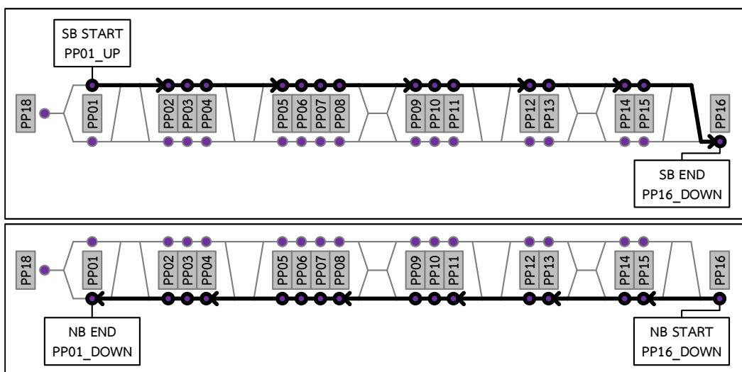
รูปที่ 1 เส้นทางรถเดินรถไฟฟ้าสายสีม่วงแบบปกติ
