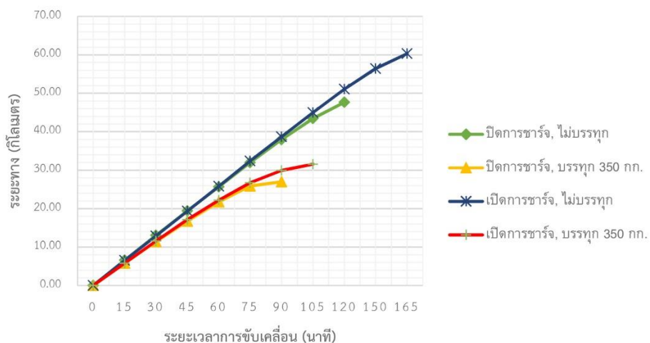
รูปที่ 5 กราฟระยะทางการขับเคลื่อนรถบรรทุกสามล้อไฟฟ้าอเนกประสงค์พลังงานแสงอาทิตย์
