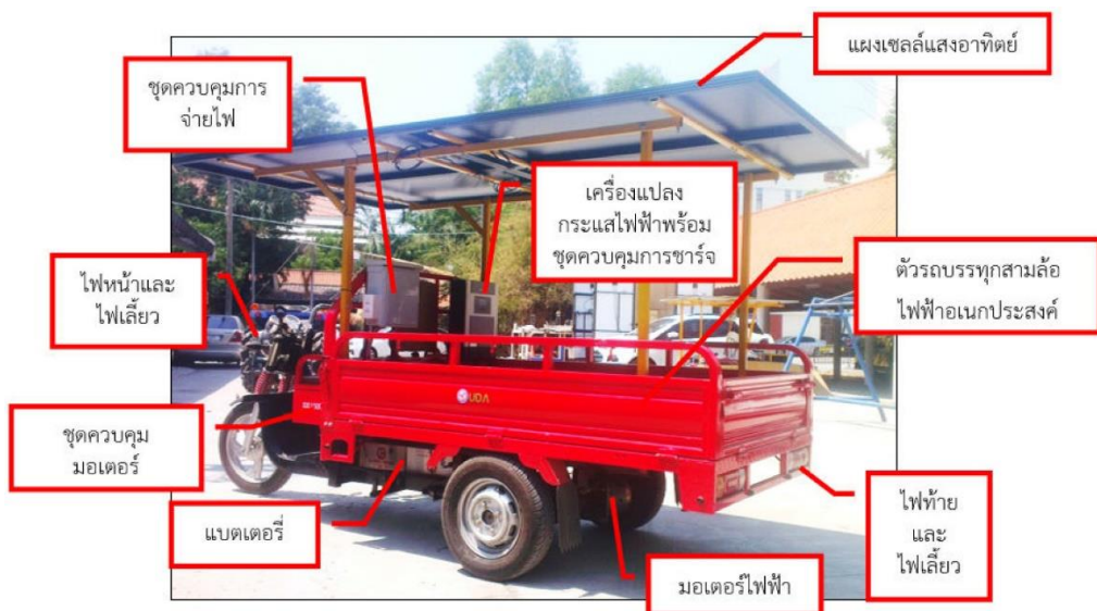
รูปที่ 2 ส่วนประกอบของรถบรรทุกสามล้อไฟฟ้าอเนกประสงค์พลังงานแสงอาทิตย์
