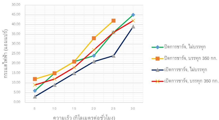
รูปที่ 4 กราฟค่ากระแสไฟฟ้าขณะขับเคลื่อนรถบรรทุกสามล้อไฟฟ้าอเนกประสงค์พลังงานแสงอาทิตย์ที่ความเร็วคงที่
