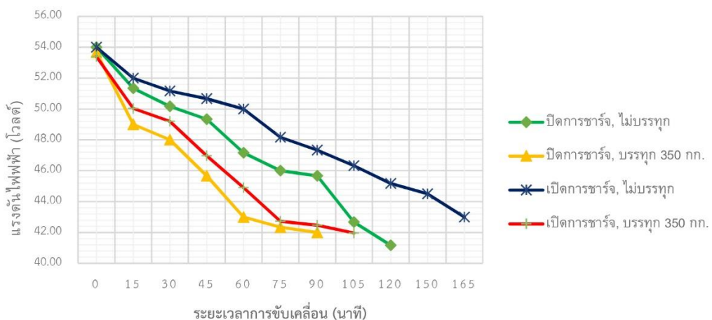
รูปที่ 8 กราฟระดับแรงดันไฟฟ้าในแบตเตอรี่ของรถบรรทุกสามล้อไฟฟ้าอเนกประสงค์พลังงานแสงอาทิตย์
