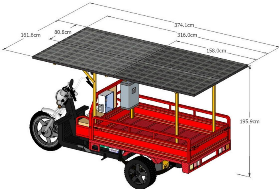
รูปที่ 1 แบบแสดงมิติของรถบรรทุกสามล้อไฟฟ้าอเนกประสงค์พลังงานแสงอาทิตย์
