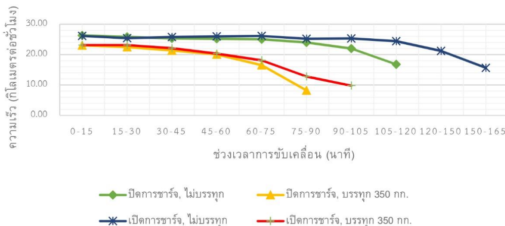
รูปที่ 6 กราฟความเร็วเฉลี่ยการขับเคลื่อนรถบรรทุกสามล้อไฟฟ้าอเนกประสงค์พลังงานแสงอาทิตย์
