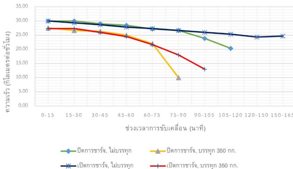
รูปที่ 7 กราฟความเร็วสูงสุดการขับเคลื่อนรถบรรทุกสามล้อไฟฟ้าอเนกประสงค์พลังงานแสงอาทิตย์
