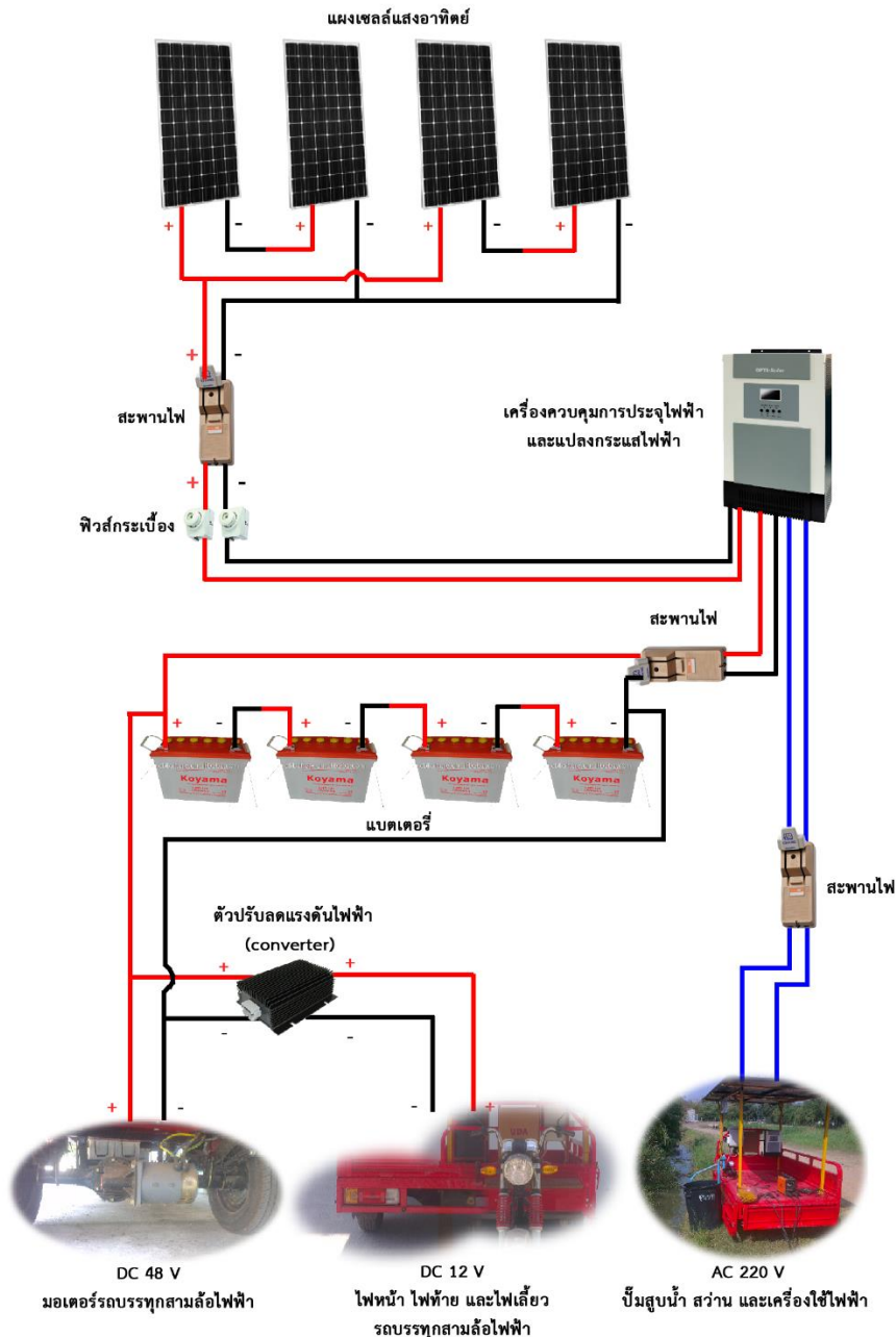
รูปที่ 3 การเชื่อมต่อระบบไฟฟ้าของรถบรรทุกสามล้อไฟฟ้าอเนกประสงค์พลังงานแสงอาทิตย์
