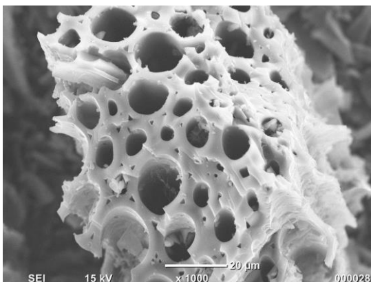
รูปที่ 3 ถ่านไผ่อายุ 12 เดือน (รูพรุนประมาณ 10 \mu\text{m} )
