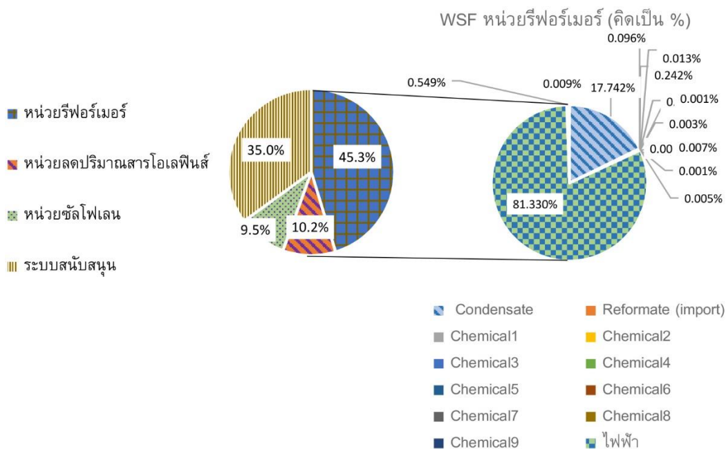
รูปที่ 7 กราฟเปรียบเทียบ WSF แยกตามกระบวนการผลิตเบนซีน
