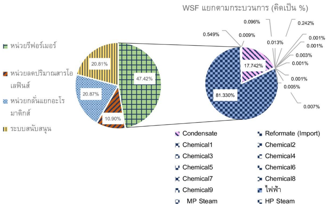
รูปที่ 8 กราฟเปรียบเทียบ WSF แยกตามกระบวนการผลิตพาราไซลีน
