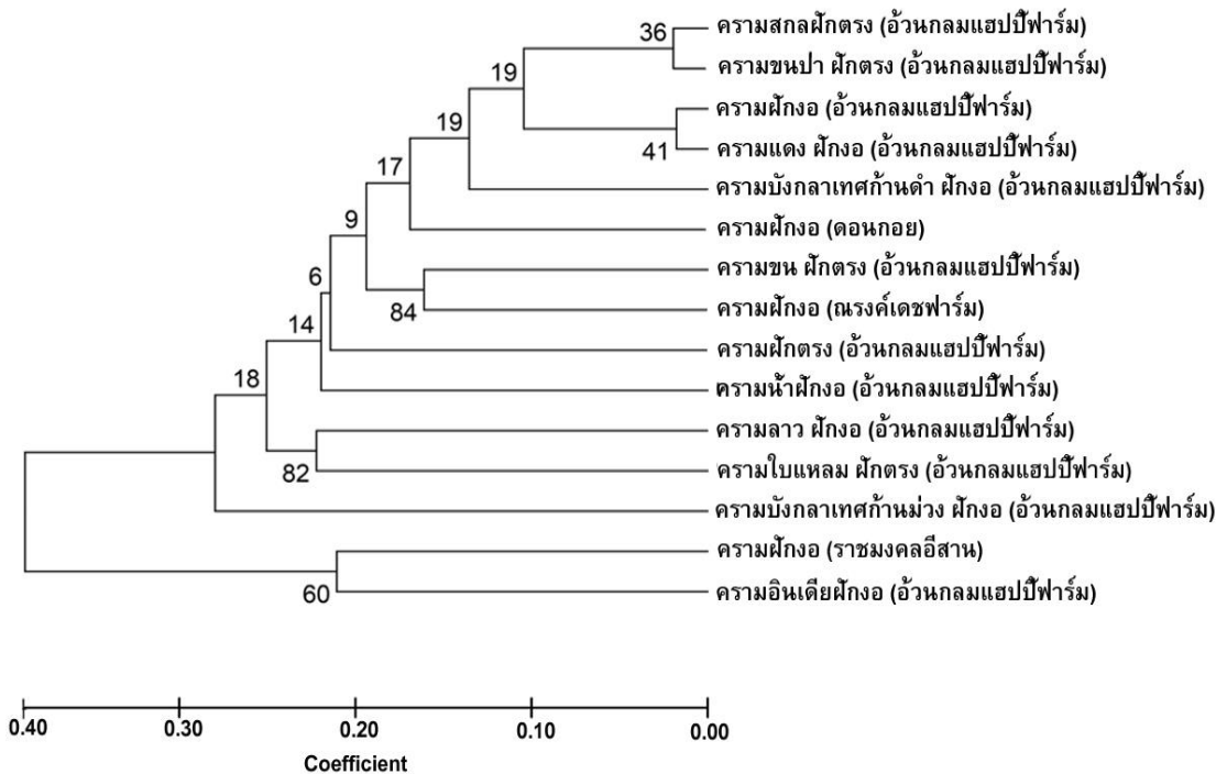
รูปที่ 1 แผนภูมิความสัมพันธ์ทางพันธุกรรมของพืชครามสกุล Indigofera ที่ได้จากลำดับนิวคลีโอไทด์ของยีน rpoC1 ซึ่งวิเคราะห์ด้วยโมเดล Tamura 3-parameter และจัดกลุ่มด้วยวิธี UPGMA
