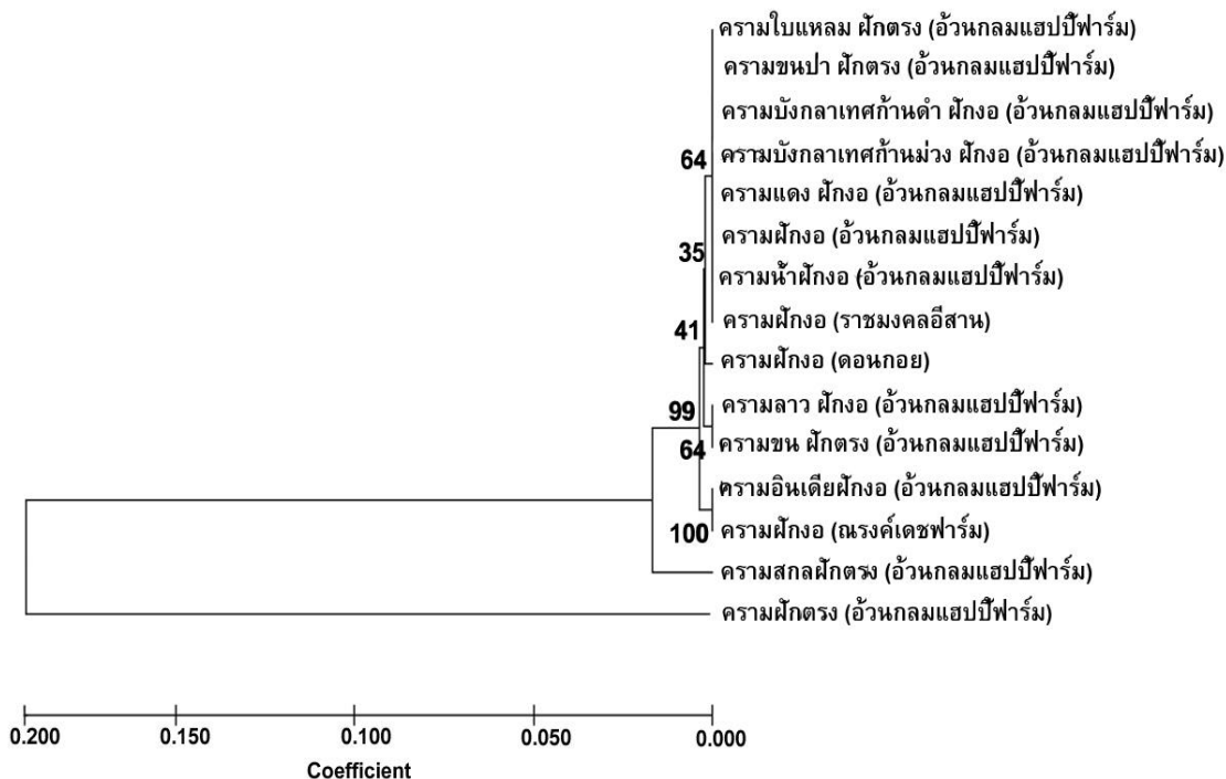
รูปที่ 2 แผนภูมิความสัมพันธ์ทางพันธุกรรมของพืชครามสกุล Indigofera ที่ได้จากลำดับนิวคลีโอไทด์ของยีน ดีเอ็นเอระหว่างยีน tmH กับ psbA ซึ่งวิเคราะห์ด้วยโมเดล Tamura 3-parameter และจัดกลุ่มด้วยวิธี UPGMA
