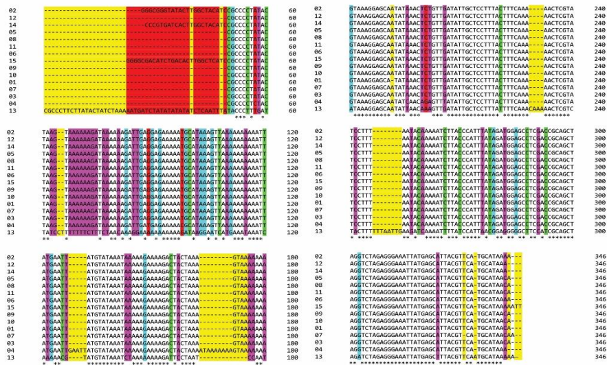
รูปที่ 4 การเปรียบเทียบนิวคลีโอไทด์ของชิ้นดีเอ็นเอระหว่งยีน trnH กับ psbA ด้วยโปรแกรม ClustalW โดยวิธี multiple alignment
