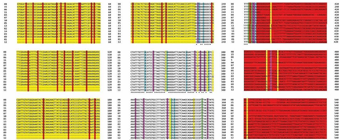
รูปที่ 3 การเปรียบเทียบลำดับนิวคลีโอไทด์ยีน rpoC1 ด้วยโปรแกรม ClustalW โดยวิธี multiple alignment
