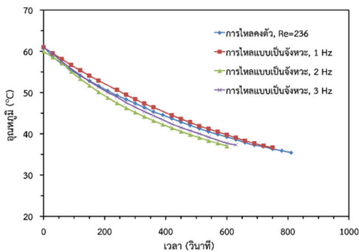
รูปที่ 6 อุณหภูมิที่กึ่งกลางไส้กรอกกับเวลากรณีการไหลแบบเป็นจังหวะไม่คงตัวที่ Re_D = 236
