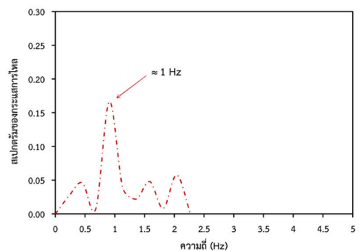
รูปที่ 4 ค่าสเปกตรัมของกระแสการไหลกับความถี่ที่ Re_D = 236
