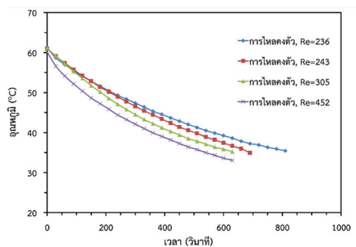
รูปที่ 5 อุณหภูมิที่กึ่งกลางไส้กรอกกับเวลาการฉีกการไหลคงตัว
