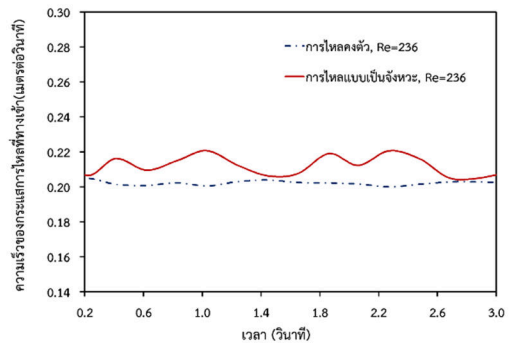
รูปที่ 3 การไหลคงตัวและการไหลแบบเป็นจังหวะไม่คงตัวที่ Re_D = 236
