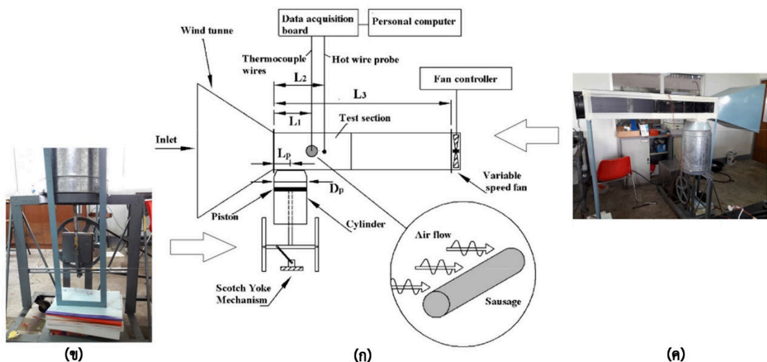
รูปที่ 2 (ก) แผนภาพชุดทดลอง (ข) ภาพถ่ายการติดตั้งกลไกสก็อตโยค และ (ค) ภาพถ่ายชุดทดลอง
