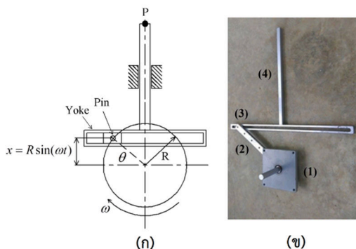
รูปที่ 1 แผนภาพและภาพถ่ายกลไก Scotch Yoke ที่ใช้ในการศึกษา
