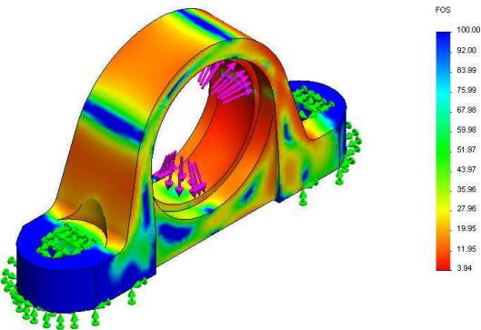
รูปที่ 10 แสดงการกระจายตัวของความเครียดและ การกระจายค่าความปลอดภัยของเสื้อลูกปืน (ที่มา: กุศล, 2553) [9]
