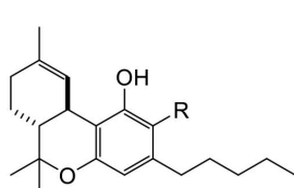
R = H : THC (1) R = CO 2 H : THCA (1a)
