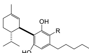
R = H : CBD (2) R = CO 2 H : CBDA (2a)
