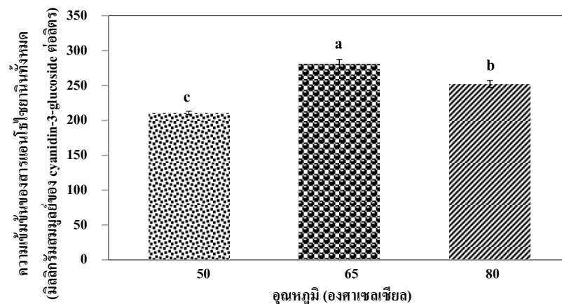
รูปที่ 3 ความเข้มข้นของสารแอนโธไซยานินทั้งหมดที่สกัดได้จากซังแห้งของข้าวโพดข้าวเหนียวสีม่วงด้วยเทคนิคการสกัดแบบอัลตราโซนิคที่อุณหภูมิ 50, 65 และ 80 องศาเซลเซียส เป็นเวลา 30 นาที และอัตราส่วนซังแห้งต่อน้ำ 1:9
