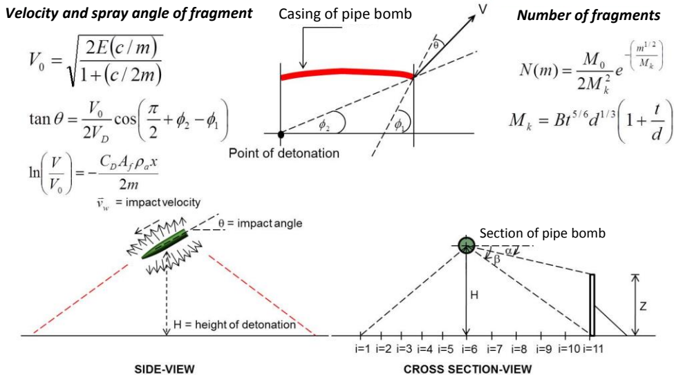
รูปที่ 6 ภาพรวมการหารัศมีการทำลายของระเบิดที่มีสะเก็ด [10]
