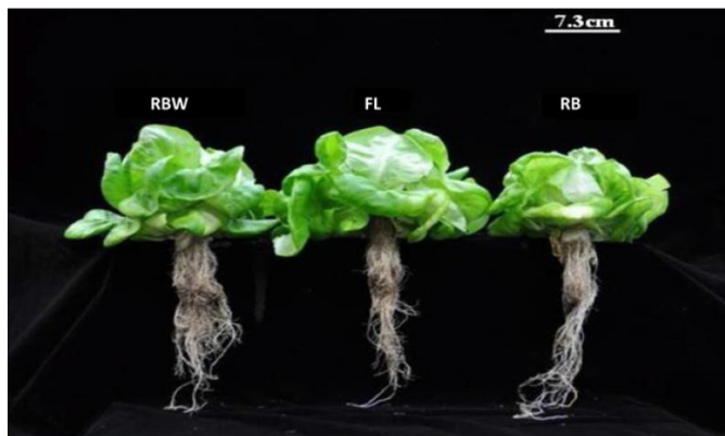
รูปที่ 8 เปรียบเทียบจำนวนราก ใบ และต้นของผักกาดหอมที่ปลูกภายใต้แสงจากไดโอดเปล่งแสงสีแดง สีนํ้าเงิน และสีขาว (RBW) และแสงจากหลอดฟลูออเรสเซนต์ (FL) และแสงจากไดโอดเปล่งแสงสีแดงและสีนํ้าเงิน (RB) แสดงในรูปที่ 8
