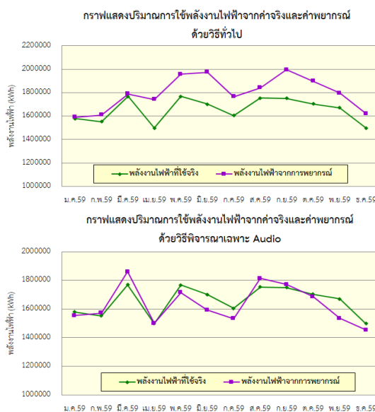
รูปที่ 5 การเปรียบเทียบผลของปริมาณการใช้พลังงานจริงและค่าพยากรณ์ด้วยวิธีต่าง ๆ
