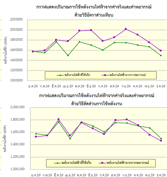
รูปที่ 5 การเปรียบเทียบผลของปริมาณการใช้พลังงานจริงและค่าพยากรณ์ด้วยวิธีต่าง ๆ
